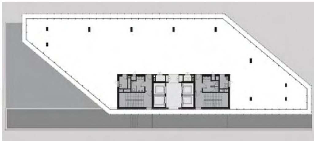
Imagen 5.24. Planta tipo.
