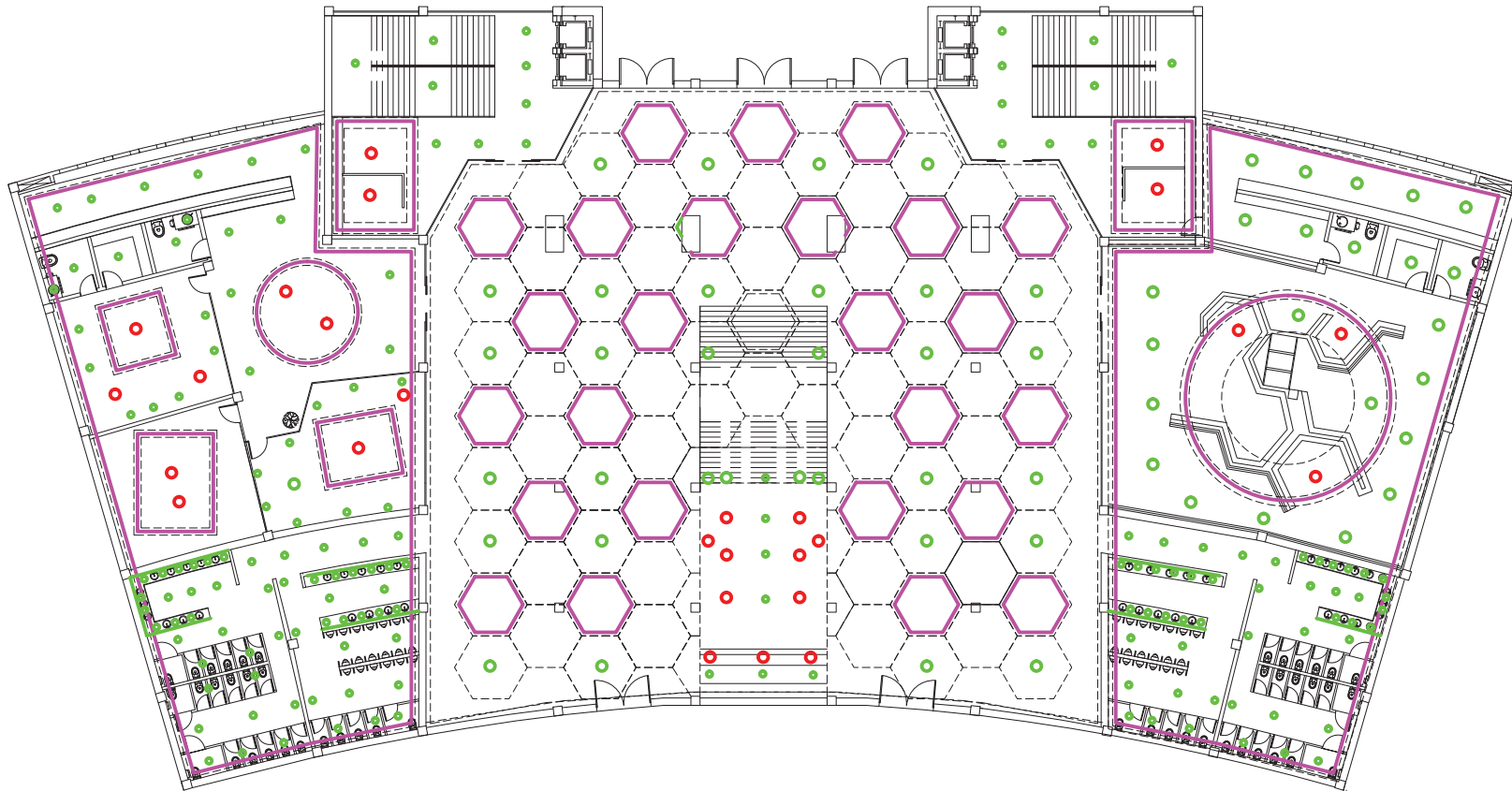
PLANTA BAJA HALL PRINCIPAL
