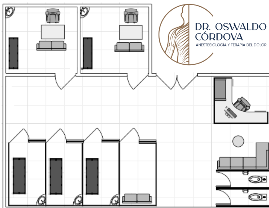
Figura 2. Diseño del “CENTRO INTEGRAL DE TERAPIA DEL DOLOR DR. OSWALDO CÓRDOVA”
