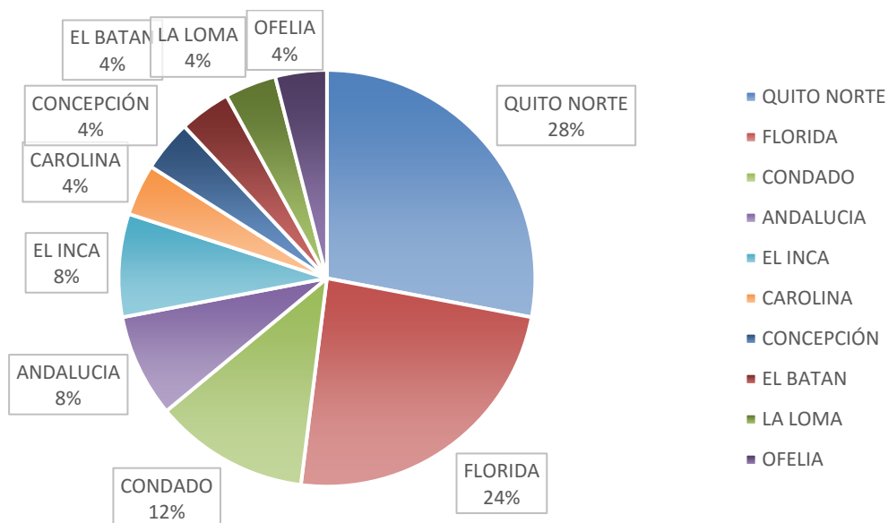
Figura 8. Pregunta 7
