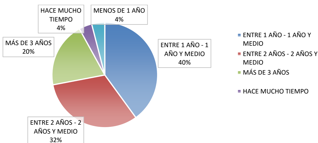
Figura 4. Pregunta 3
