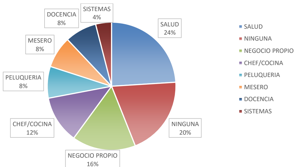
Figura 6. Pregunta 5
