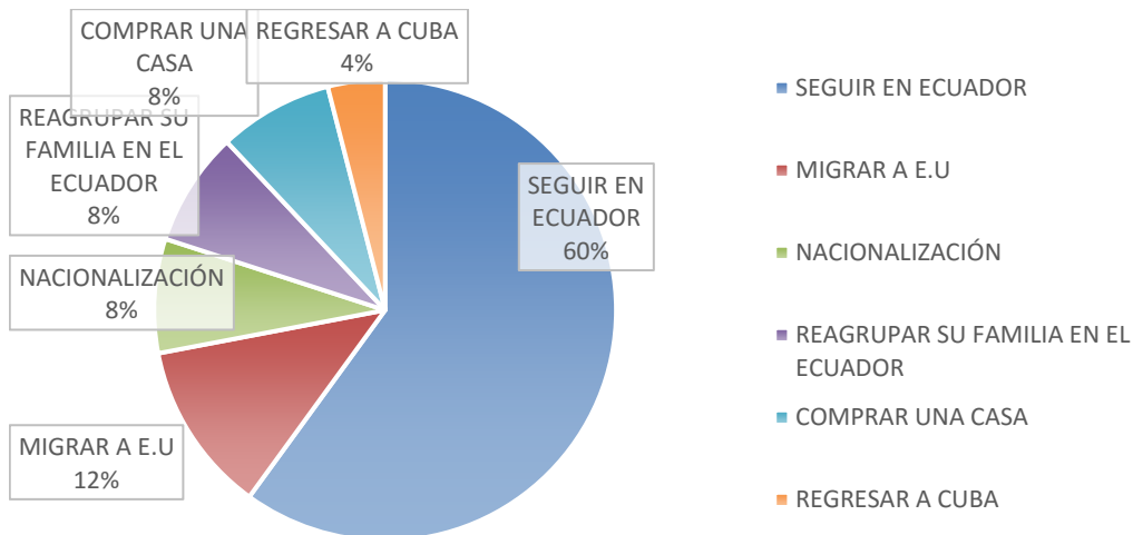
Figura 9. Pregunta 8
