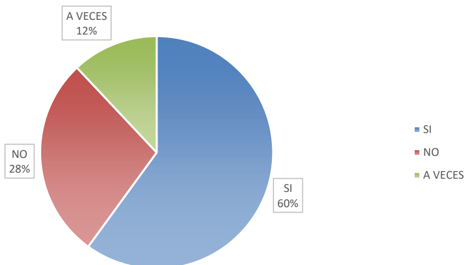
Figura 13. Pregunta 12
