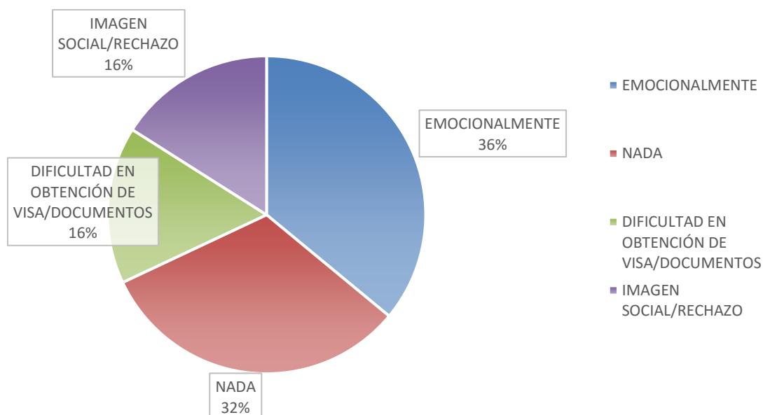
Figura 7. Pregunta 6
