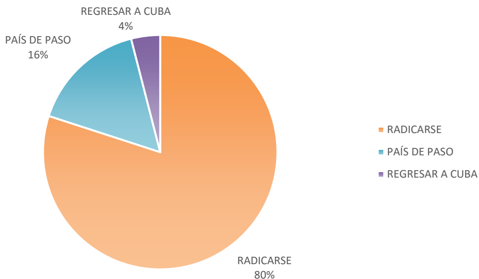
Figura 10. Pregunta 9
