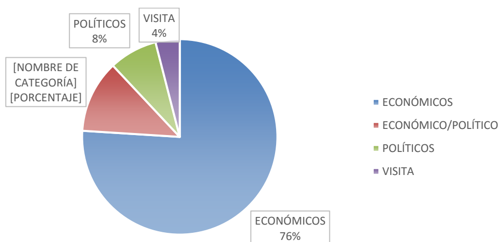
Figura 2. Pregunta 1
