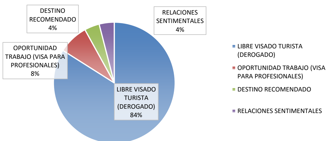
Figura 3. Pregunta 2
